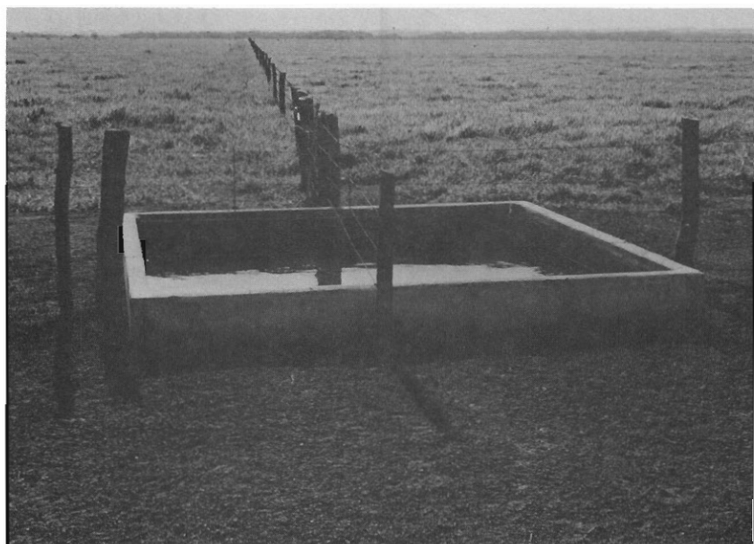
Figura 11. Bebedero-tanque construido en la intersección de varios potreros.
