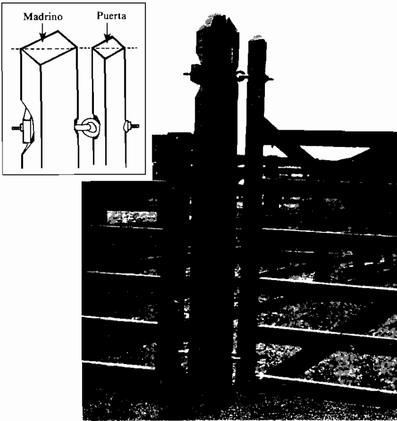
Figura 20. Para permitir que las puertas abran al máximo en los dos sentidos, las aristas del madriño y de la puerta que llevan los goznes deben quedar frente a frente.
