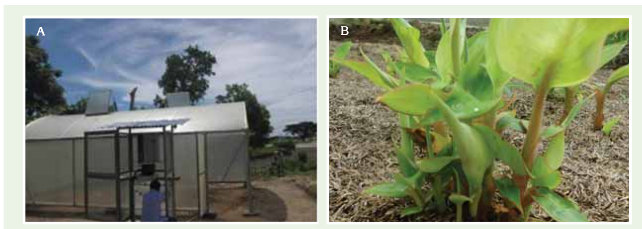
Figura 13. Sistema de propagación masiva de semilla limpia, en cámara térmica.
