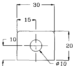
Detalle A
