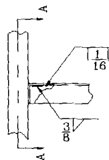
Detalle C
