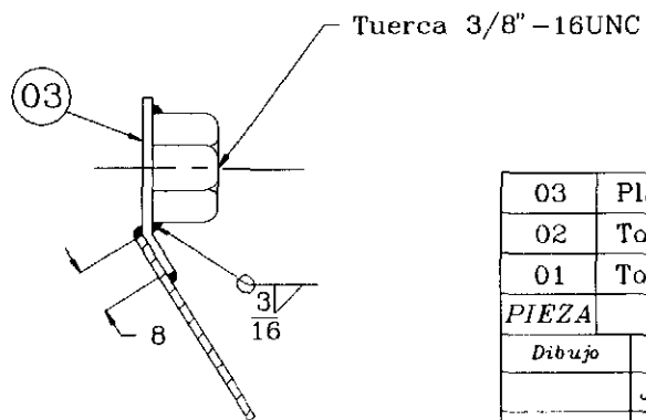
Detalle B
