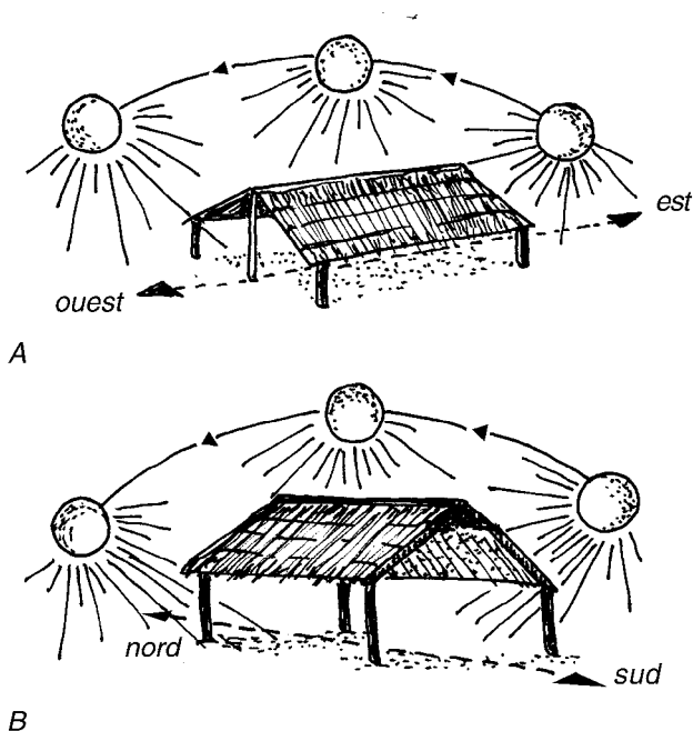
Figure 14: A : chèvrerie orientée selon un axe est-ouest B : chèvrerie orientée selon un axe nord-sud
