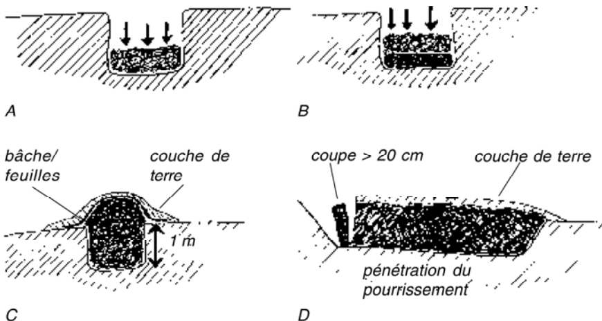
Figure 11: A : On met en place la première couche et on la tasse B : On ajoute une deuxième couche sur la première et on la tasse également.
